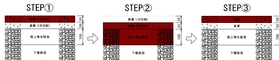
施工断面図
