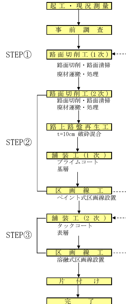
(a) 施工手順 施工フロー(車道)
